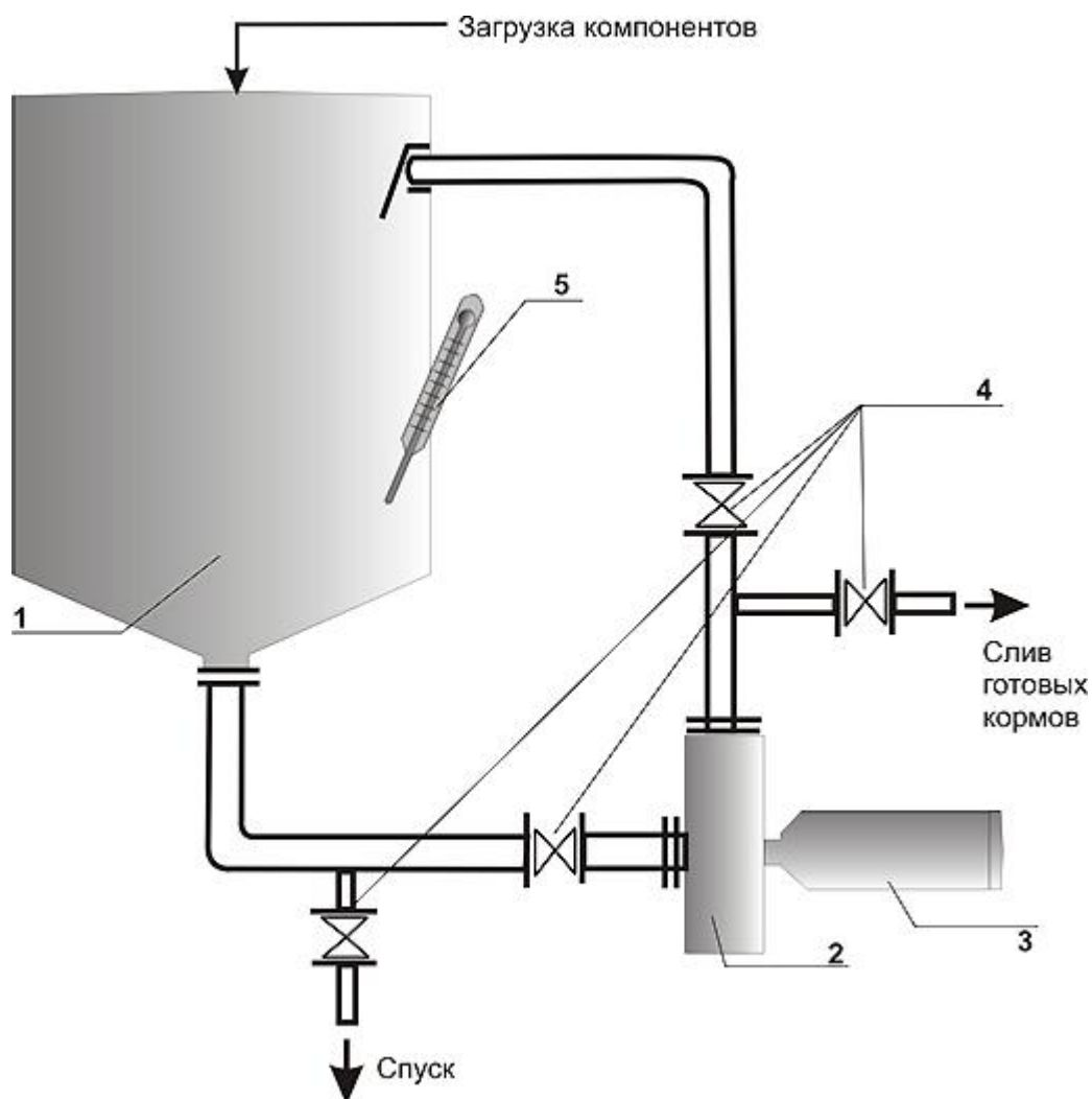
1–Рабочий бак; 2–Диспергатор; 3–Электродвигатель; 4–Поворотные клапаны; 5–Термометр
